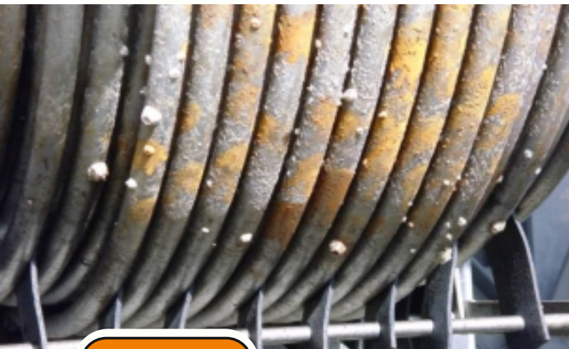
Усунення накипу від морської води та мікроорганізмів
