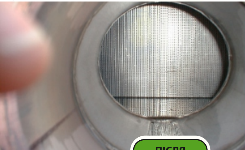
Усунення гематиту з компактного теплообмінника
